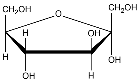
\alpha -fructose
