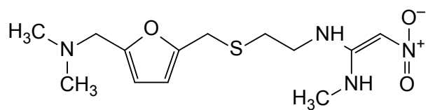
ranitidine
