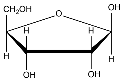
ribose
